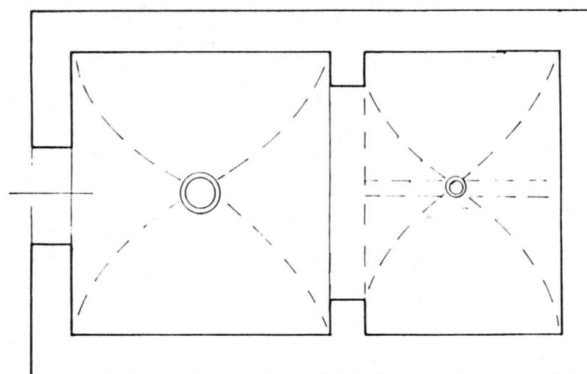
Chiesa della masseria "Grottone". Pianta.
