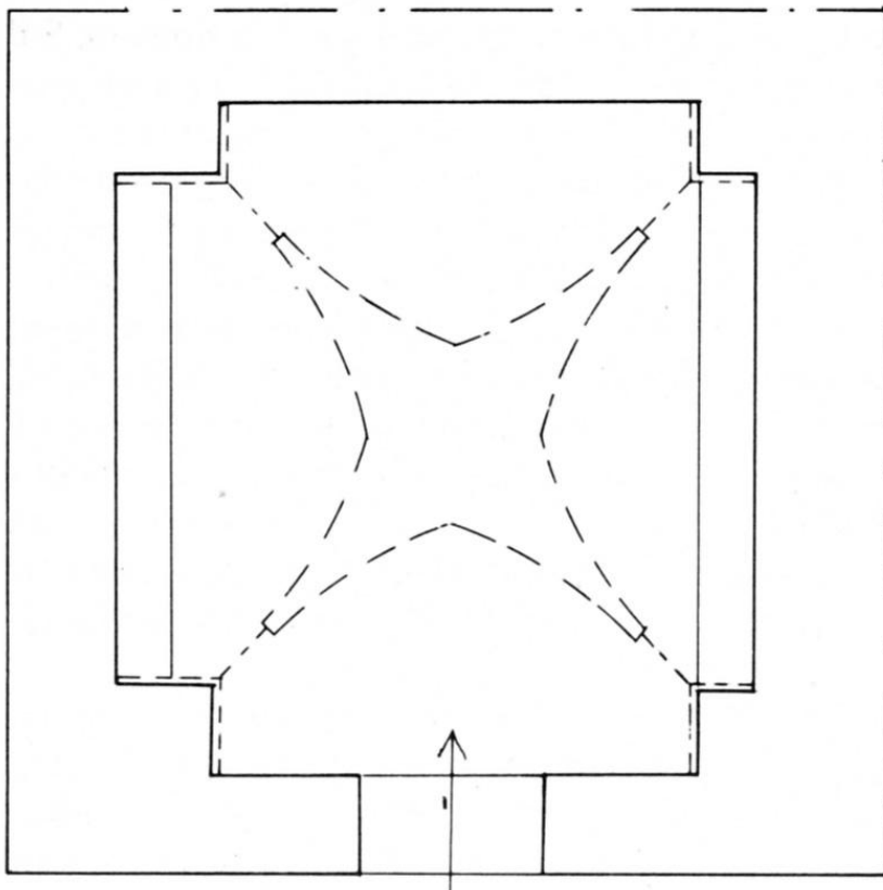
Chiesa della masseria "Giovannarola". Pianta.
