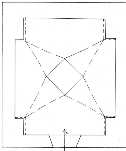
Chiesa "Camillo Tanzarella". Pianta.
